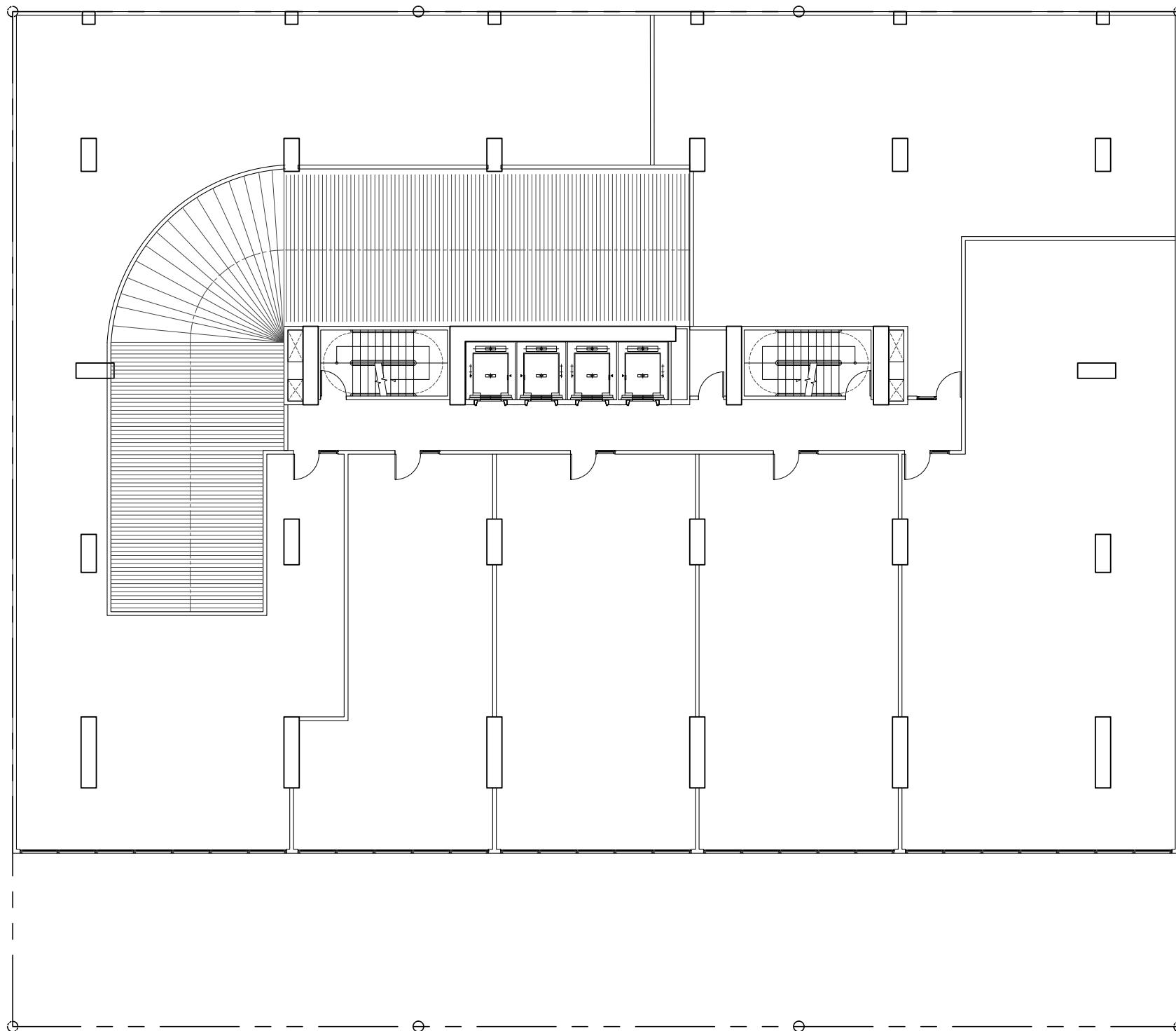
PLANTA NIVEL 100
