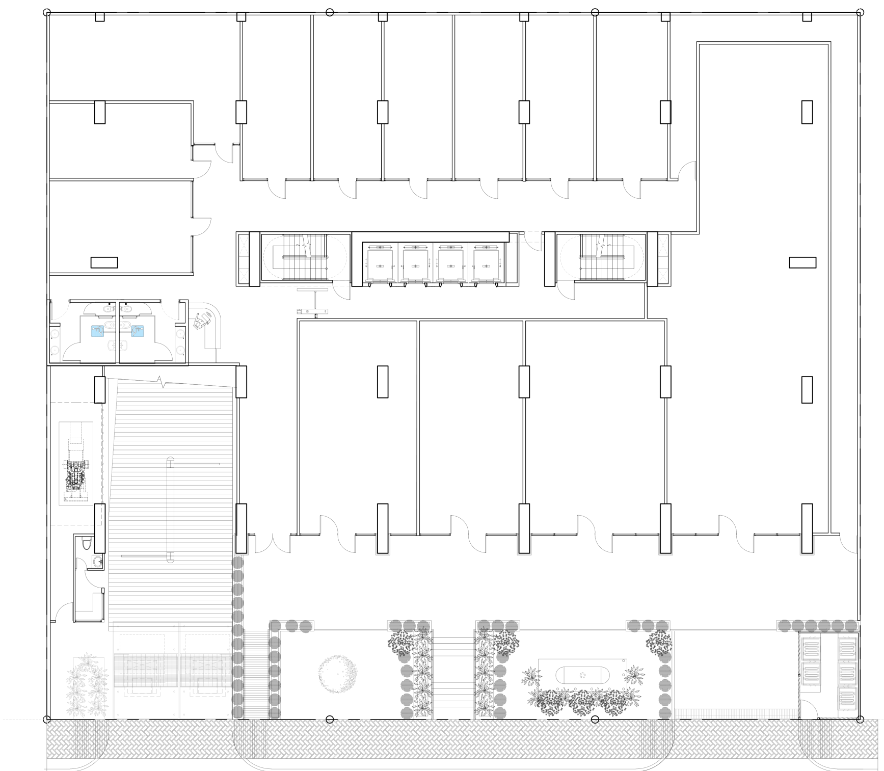
PLANTA BAJA
